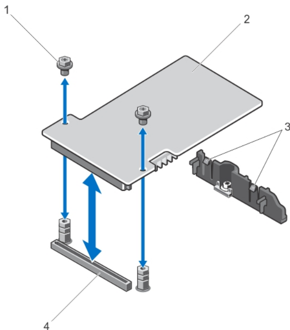
图 24: 卸下和安装存储控制器卡
