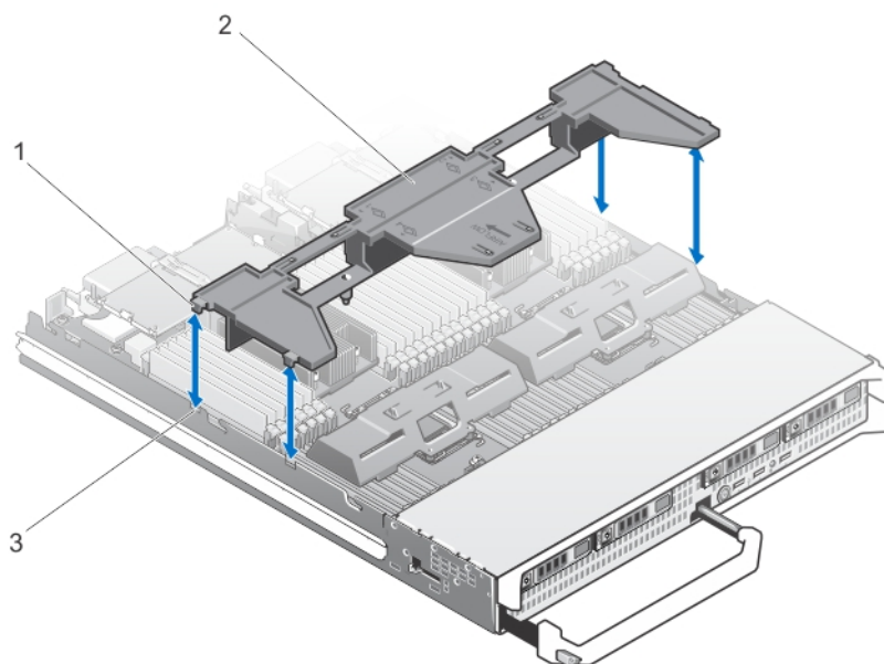
图 6: 卸下和安装冷却导流罩
