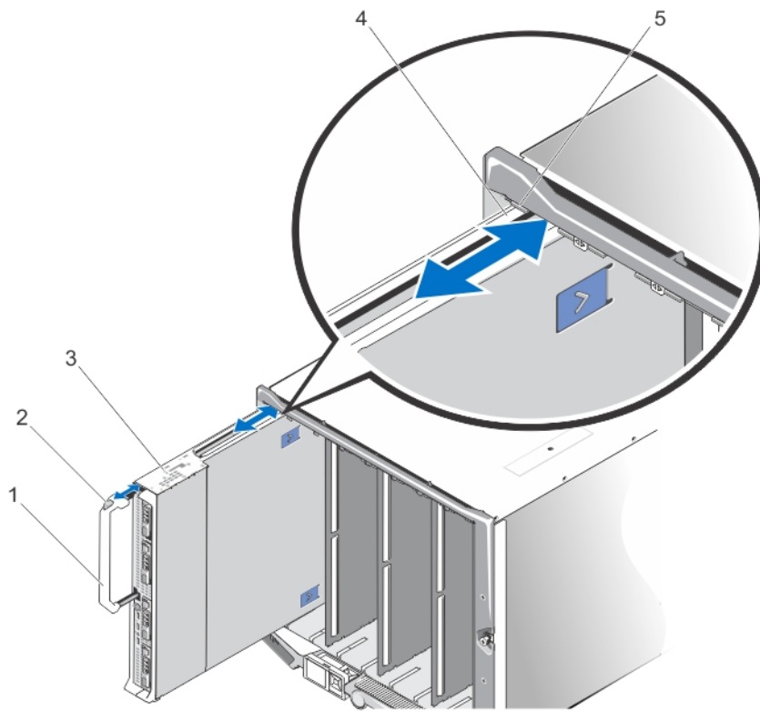
图 3: 卸下和安装刀片
