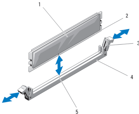
图 22: 安装和卸下内存模块或内存模块挡板
