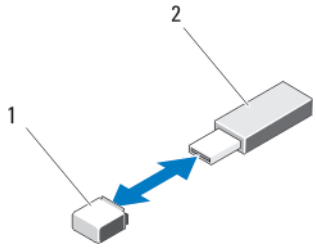
图 14: 装回 USB 存储钥匙
