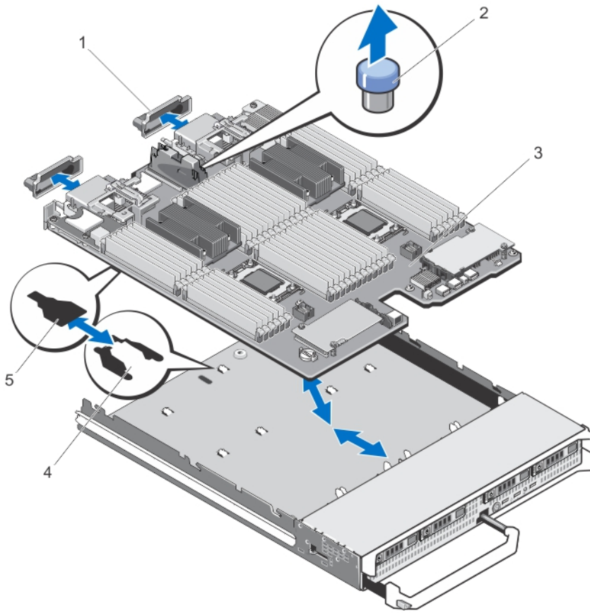
图 20: 卸下和安装系统板
