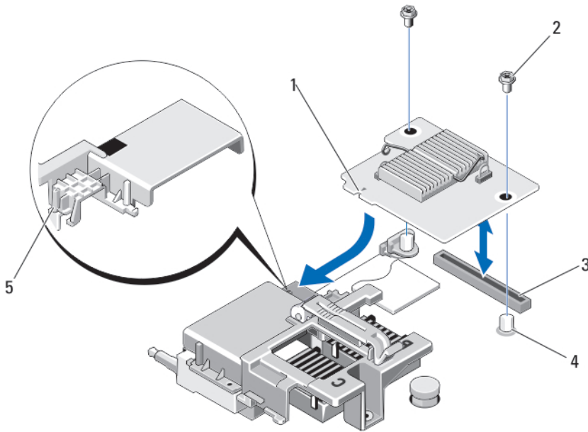
图 12: 卸下和安装网络子卡/LOM 提升卡
