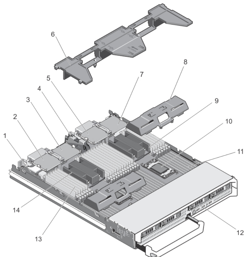
图 5: 刀片内部
