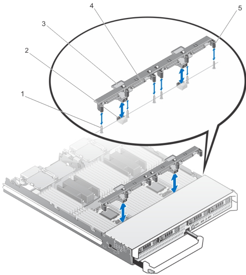
图 9: 卸下和安装硬盘驱动器/SSD 背板 (全长)
