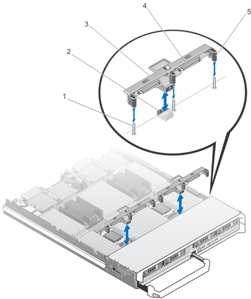
图 10: 卸下和安装硬盘驱动器/SSD 背板（半长）
