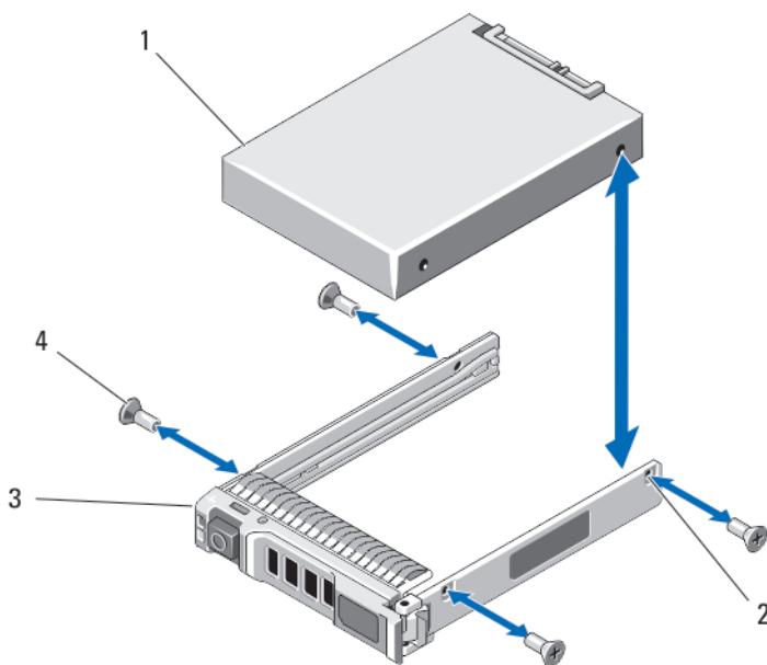
图 8: 在硬盘驱动器/PCIe SSD 托盘中卸下和安装硬盘驱动器/PCIe SSD
