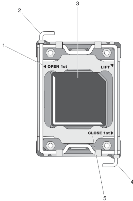
图 18: 处理器护盖打开与合上拉杆的顺序
