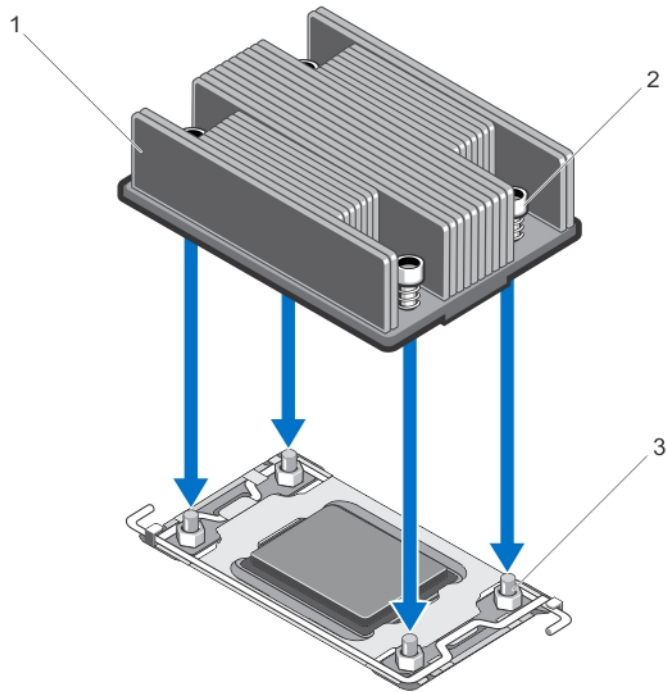
图 17: 卸下和安装散热器
