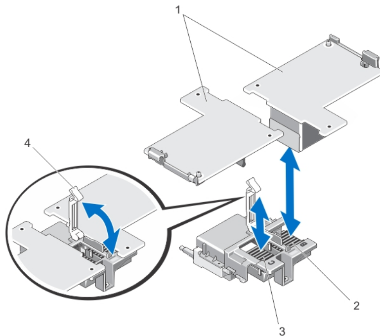
图 11: 卸下和安装夹层卡
