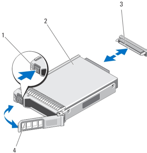
图 7: 卸下和安装硬盘驱动器/PCIe SSD
