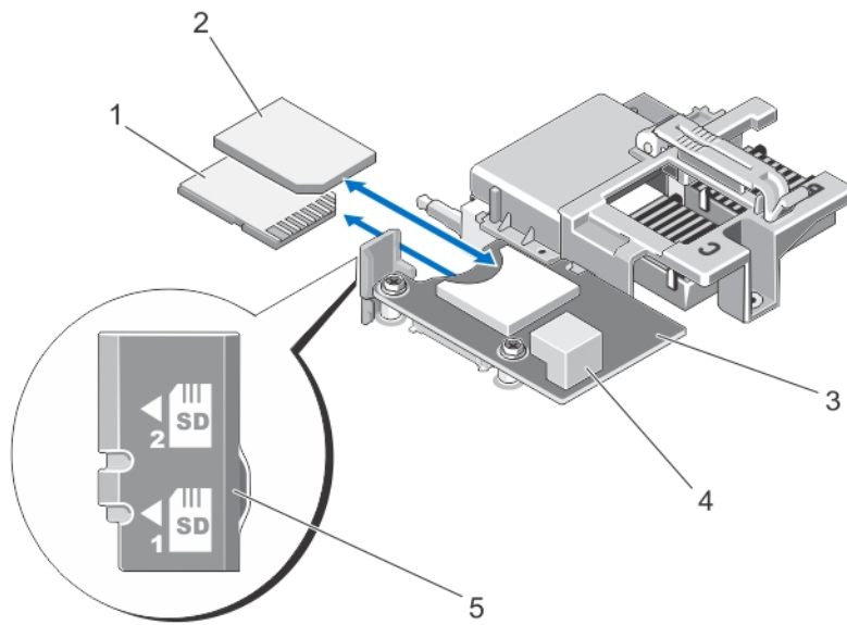
图 13: 更换 SD 卡
