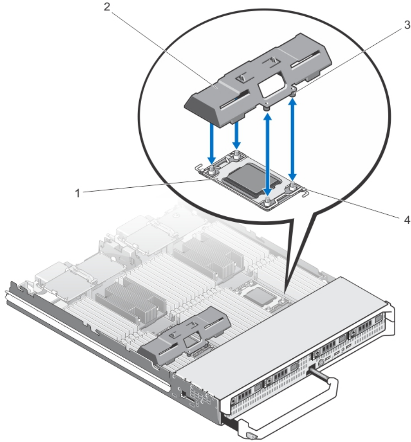
图 16: 卸下和安装处理器/DIMM 挡板
